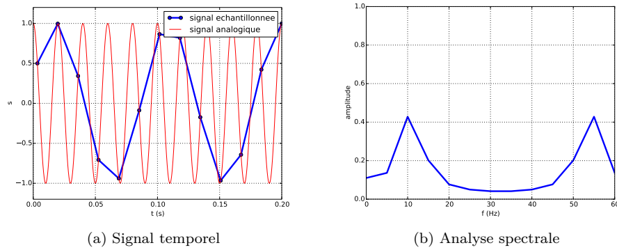
FIGURE 6 – Signal insuffisamment échantillonné : f = 50 \text{ Hz} et f_e = 60 \text{ Hz}
