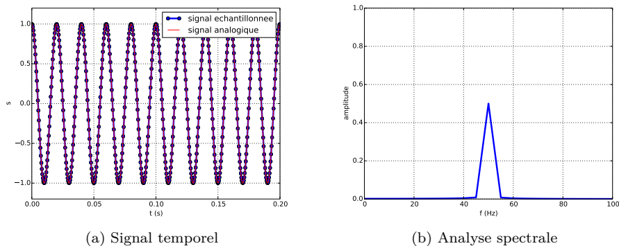
FIGURE 4 – Signal très bien échantillonné : f = 50\text{ Hz} et f_e = 2500\text{ Hz} .
