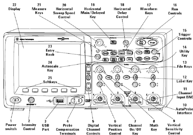
FIGURE 1 – Interface d'un oscilloscope numérique
