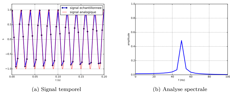
FIGURE 5 – Signal correctement échantillonné : f = 50\text{ Hz} et f_e = 250\text{ Hz} .
